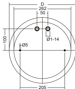
D 370/420
