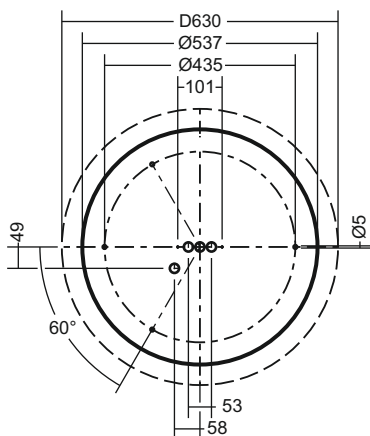
D 630
