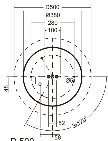
D 500
