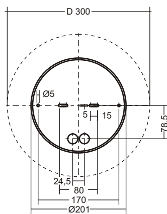
D 300
