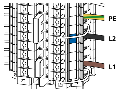
1-phasiger Anschluss (IT Netz) der Versorgungsleitung (230 V)
