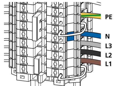
3-phasiger Anschluss der Versorgungsleitung (400 V)
