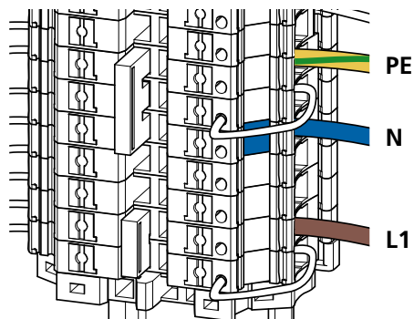
Syöttökaapelin yksivaiheiliitäntä (400 V) 1-fasanslutning vid 230V
