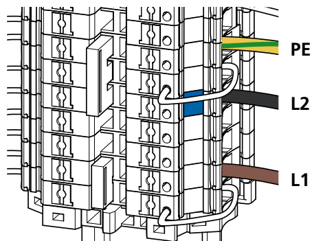
1-vaiheinen liitäntä (IT-verkko) syöttöjohto (230 V) 1-fasanslutning (IT-nätverk) matningsledningen (230 V)
