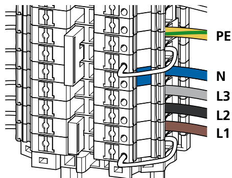
Syöttökaapelin kolmivaiheiliitäntä (400 V) 3-fasanslutning vid 400V
