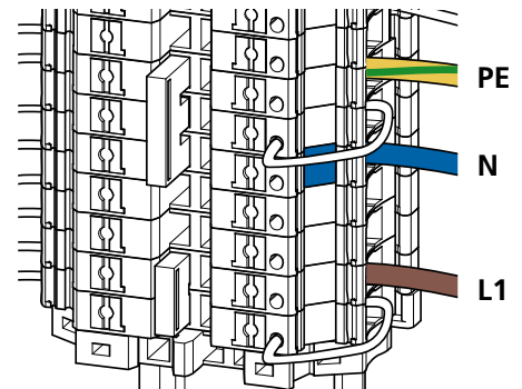
1-phasiger Anschluss der Versorgungsleitung (230 V)
